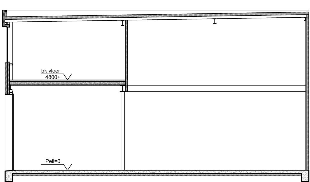
Doorsnede
