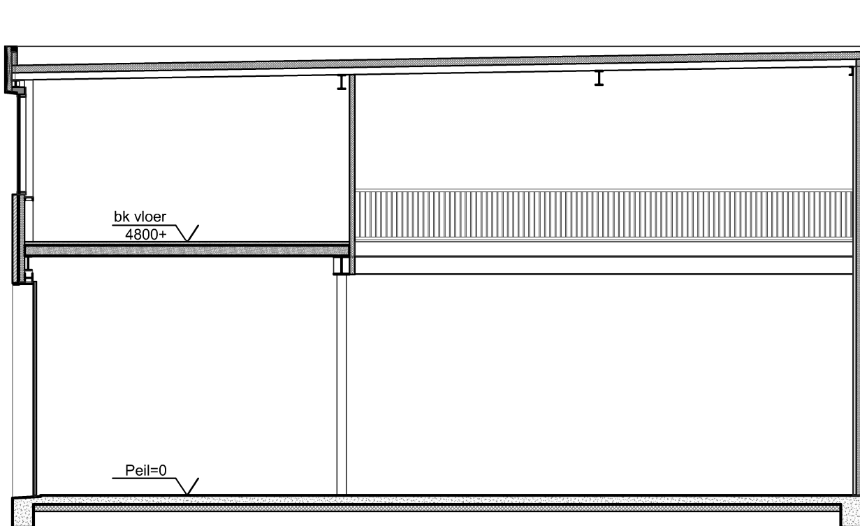
Doorsnede
